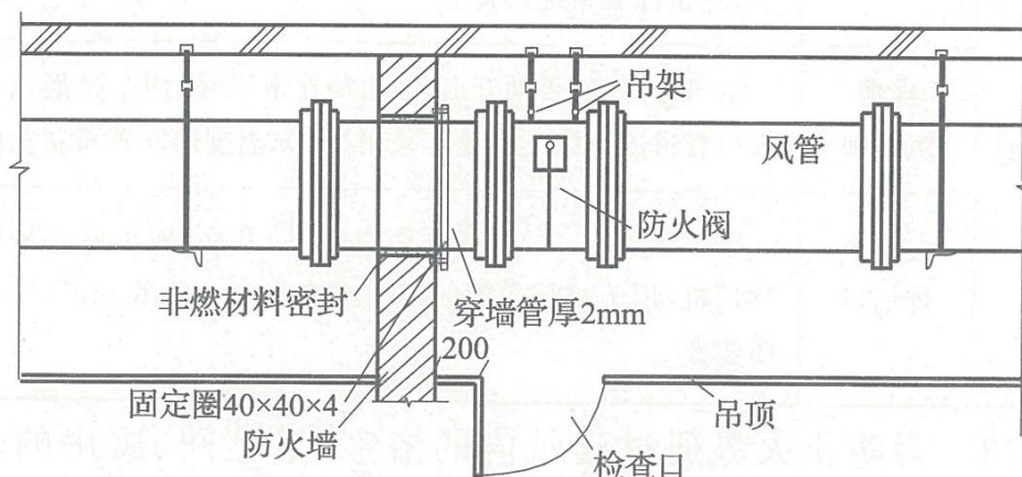
图 10 防火阀检修口设置示意图
