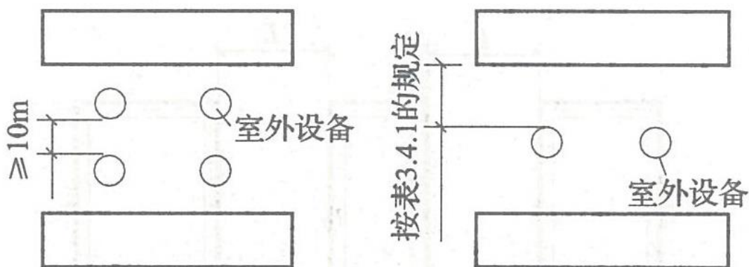
图 1 有室外设备时的防火间距
