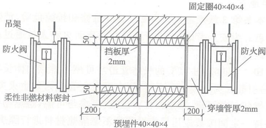
图 9 变形缝处的防火阀
