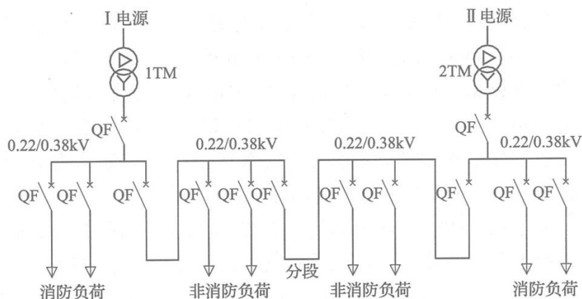
负荷不分组设计方案（二）
