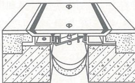
图7 变形缝构造示意图
