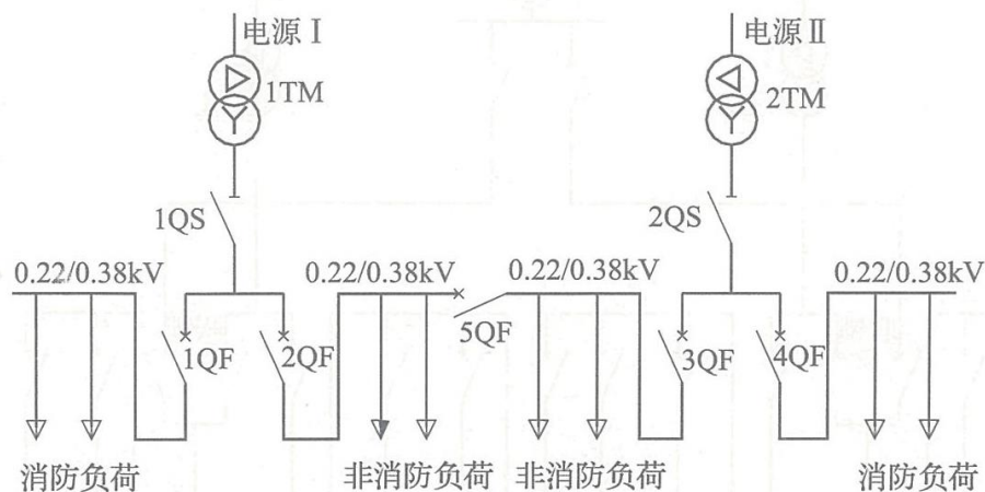
负荷分组设计方案（一）
