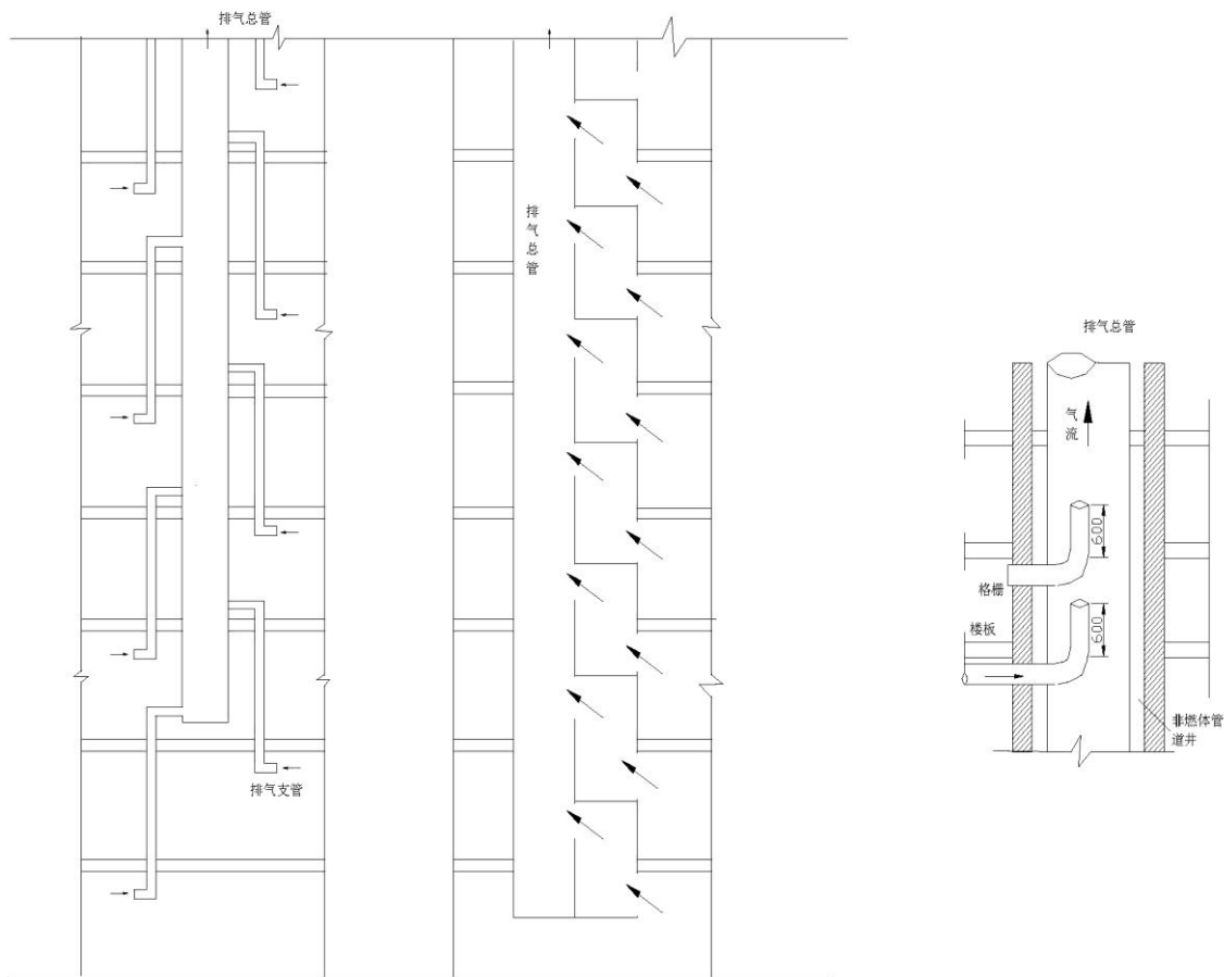
图8 排气管防止回流示意图
