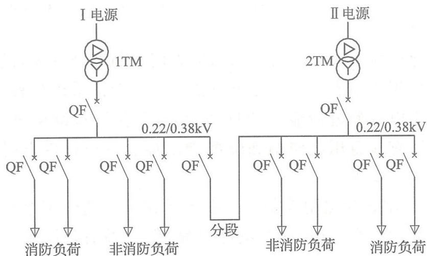
负荷不分组设计方案（一）
