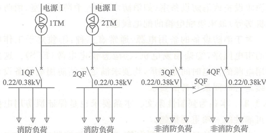
负荷分组设计方案（二）
